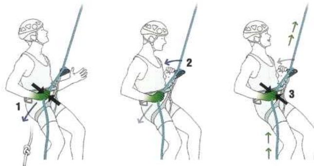
그리그리를 사용할 때 아래 손은 항상 로프를 잡고 있어야 한다.
