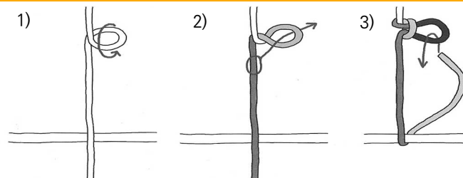
[그림 3-56] 당김줄매듭을 이용하여 로프를 당기는 방법
