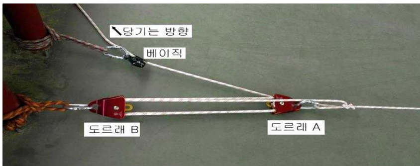
[그림 3-61] 2단 도르래를 이용한 로프 연장 방법
