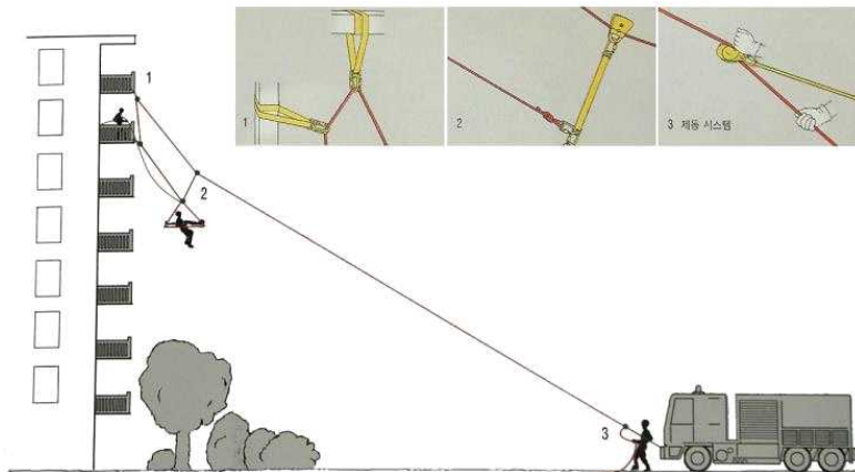
[그림 4-16] 경사하강으로 구조하기
