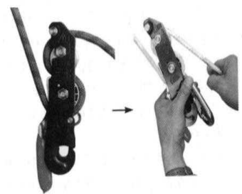
[그림 2-8] 스톱 하강기 사용법
