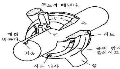
[그림 5-9] 키와 나사로 고정된 축의 분해방법
