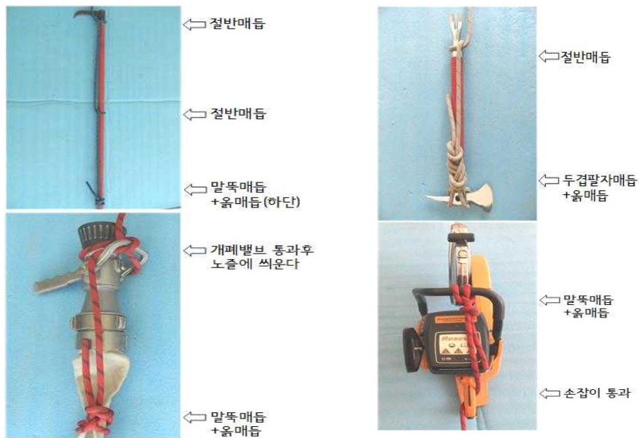
[그림 3-29] 여러가지 기구 묶기
