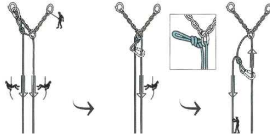
[그림 3-53] 회수 로프 설치방법
