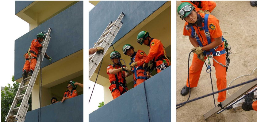
[그림 4-18] 가로대 위로 로프를 빼 내어 안전벨트에 결착
