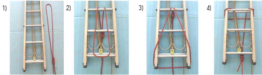
[그림 3-30] 사다리 묶기
