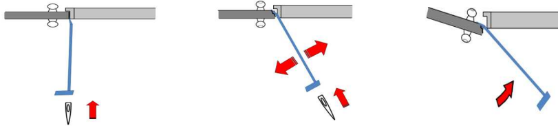
[그림 6-23] 지렛대 활용 작업(3)
