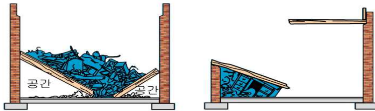
[그림 5-88] V자형 붕괴(좌)와 캔틸레버형 붕괴
