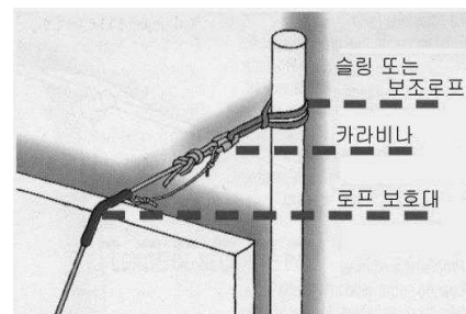
[그림 3-50] 현수로프의 간접 고정
