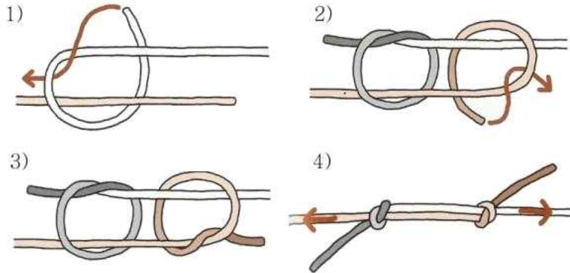
[그림 3-17] 피셔맨 매듭
