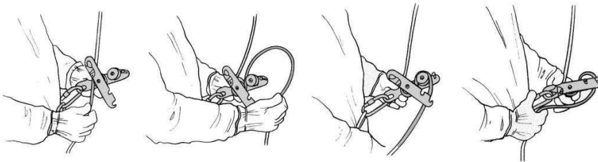
[그림 3-75] 스톱 하강기에 로프 삽입하기
