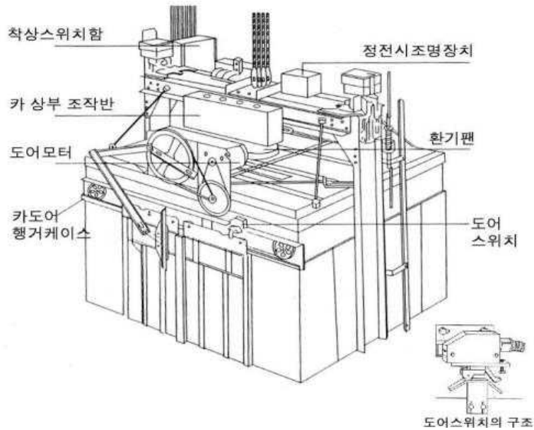
[그림 5-101] 카상부의 구조
