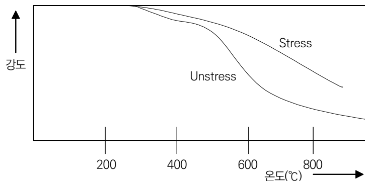
[그림 5-83] 콘크리트의 온도변화에 따른 강도 변화
