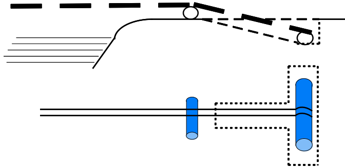
[그림 3-43] 확보물을 매몰시켜 로프를 설치하는 방법
