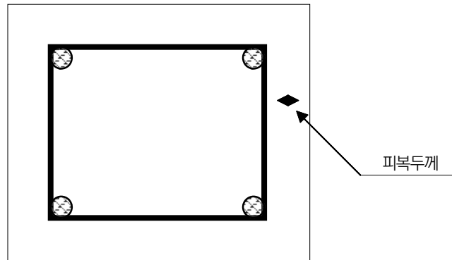
[그림 5-84] 철근 콘크리트 기둥의 단면도
