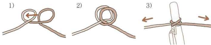
[그림 3-20] 말뚝 매기의 다른 방법, 로프 끝을 둥글게 겹쳐서 끼운다.
