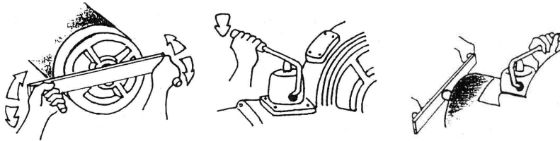
터닝 핸들과 브레이크의 조작방법 브레이크는 슈브 반대쪽에서 개방한다.
