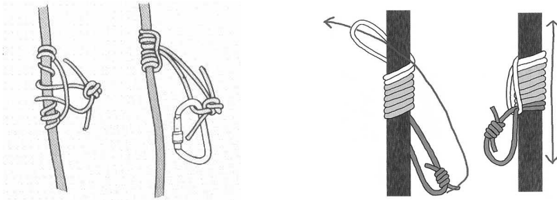
[그림 3-24] 감아매기(좌)와 클램하이스트 매듭(우)
