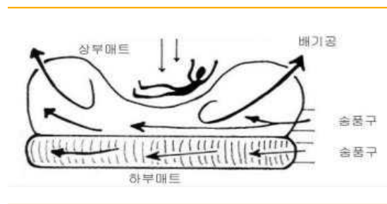
[그림 2-39] 공기매트의 구조
