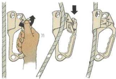
[그림 2-11] 등강기 사용방법
