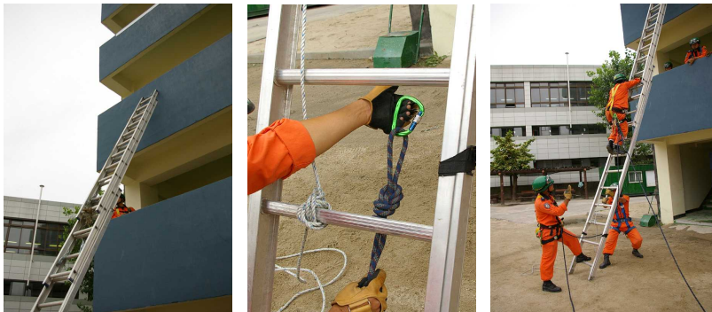
[그림 4-17] 사다리에 로프설치
