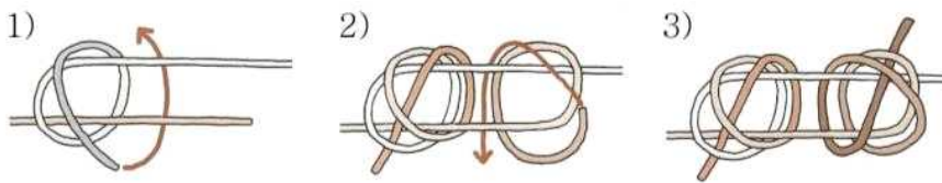
[그림 3-18] 이중 피셔맨 매듭
