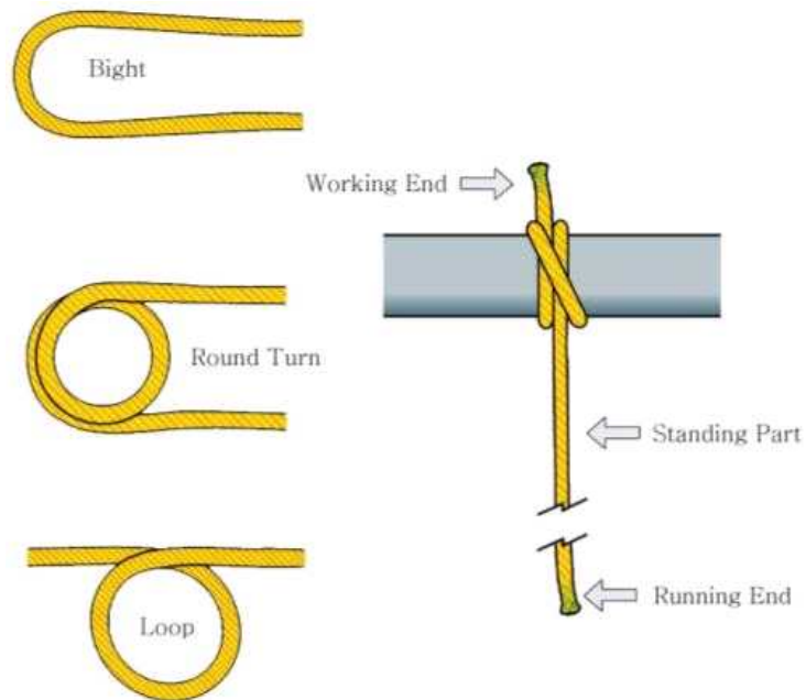
[그림 3-1] 매듭 각 부분의 명칭
