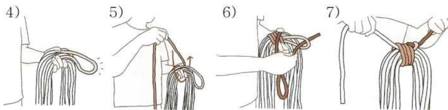
[그림 3-32] 한발감기
