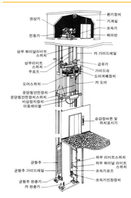
[그림 5-100] 엘리베이터의 구조
