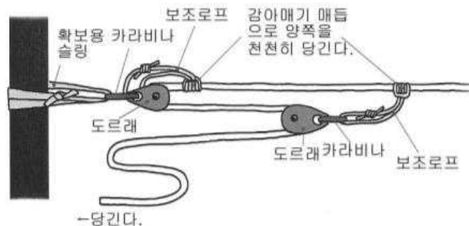
[그림 3-60] Z자형 도르래 배치법을 응용한 로프 연장법
