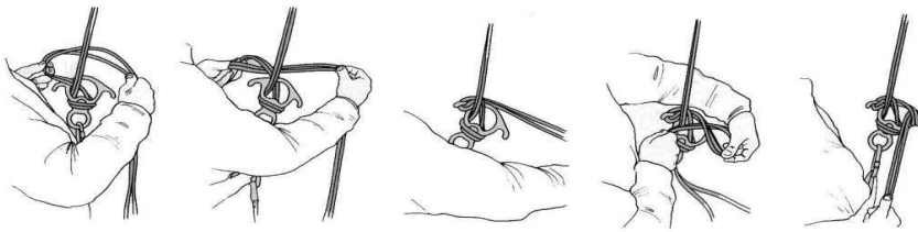
[그림 3-80] 구조용 하강기를 고정하는 방법
