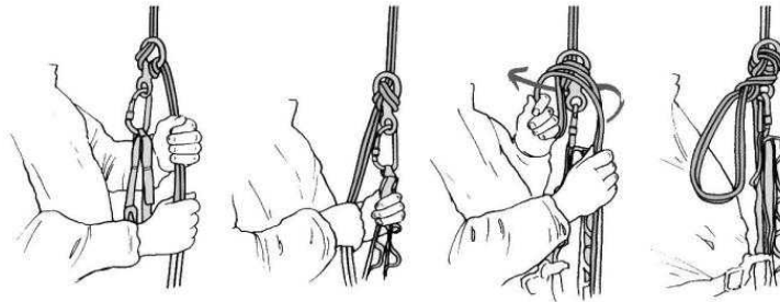
[그림 3-79] 8자 하강기를 완전히 고정하는 방법
