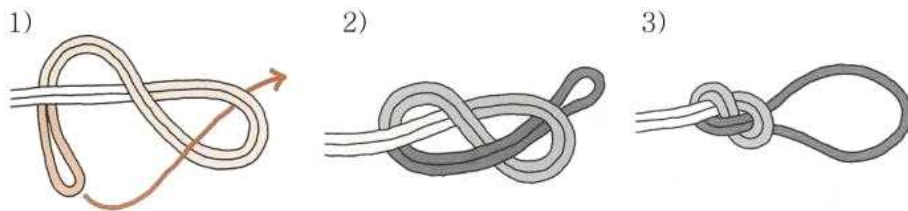
[그림 3-6] 두 겹 8자 매듭
