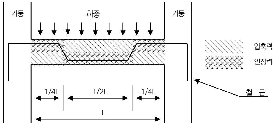
[그림 5-82] 보의 응력 분포
