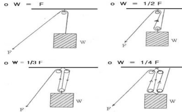
[그림 2-13] 도르래 숫자와 힘의 이득 관계
