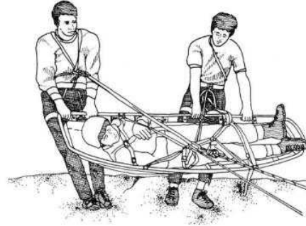
[그림 5-114] 1줄 로프로 하강하기
