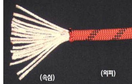
[그림 2-3] 컨먼틀 로프의 구조
