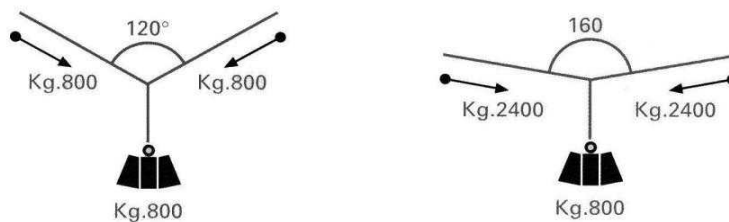
[그림 3-55] 수평으로 연장된 로프에 가해지는 장력
