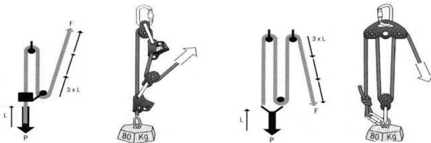
[그림 2-14] 도르래 설치방법의 예
