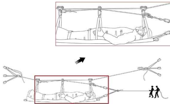
[그림 4-23] 들것을 이용한 구조대상자의 구출
