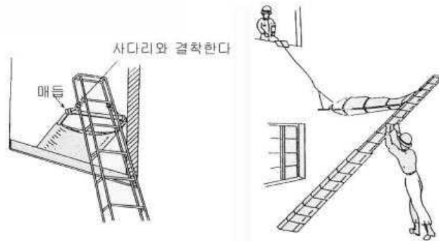
[그림 4-21] 사다리를 이용한 수평구출 방법
