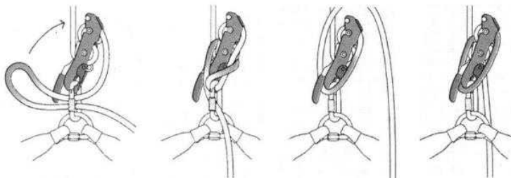
[그림 3-81] 스톱하강기 고정법
