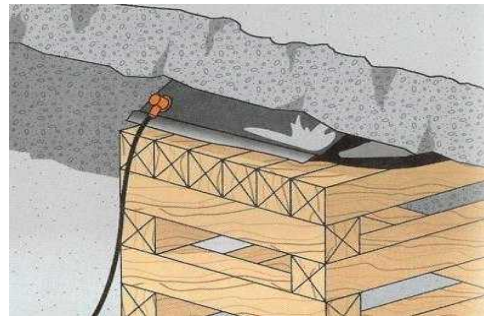
[그림 2-29] 받침목을 이용한다.
