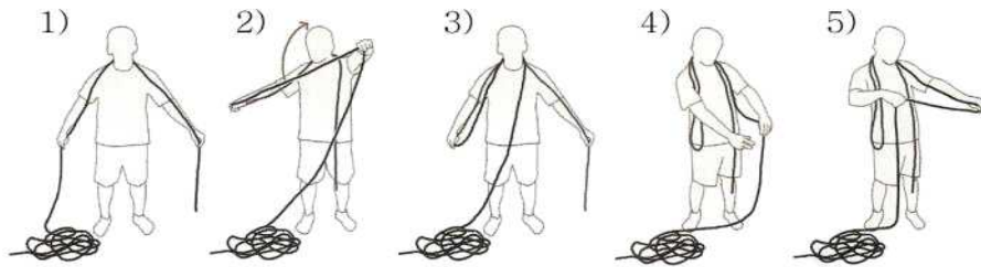
[그림 3-34] 어깨감기
