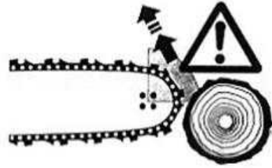
[그림 2-24] Kick Back 현상
